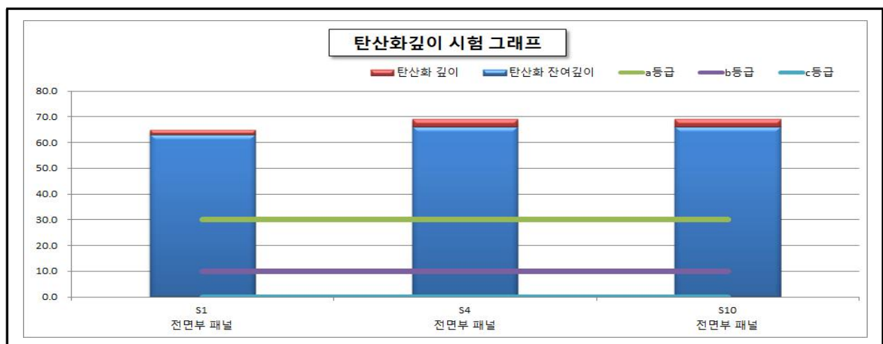
【그림 81.8】 탄산화 깊이 측정결과
