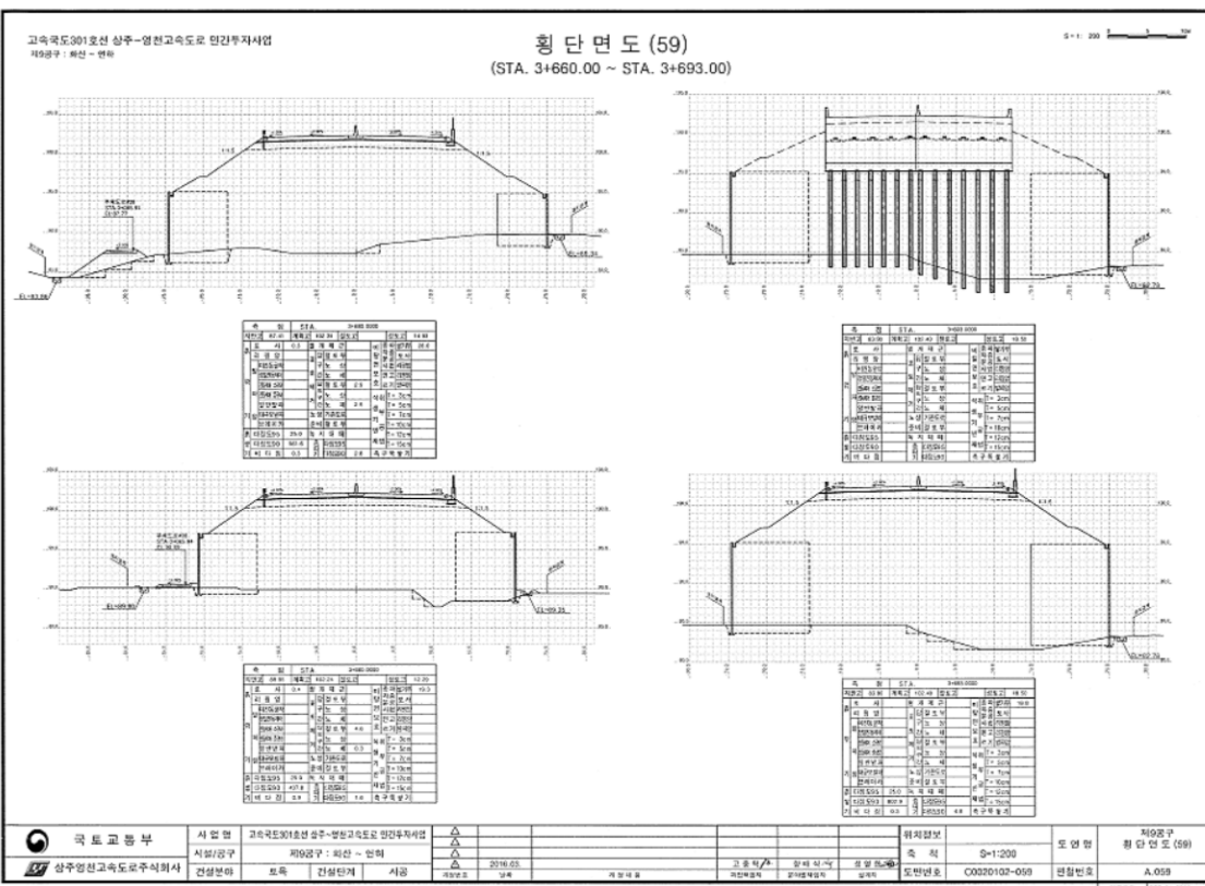
【그림 81.5】 단면도
