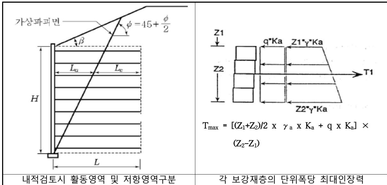
【그림 81.12】 토압작용 모식도
