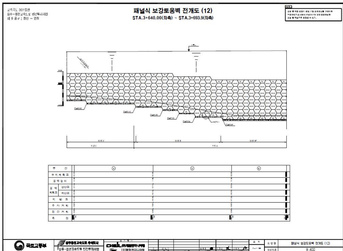
【그림 81.4】 전개도
