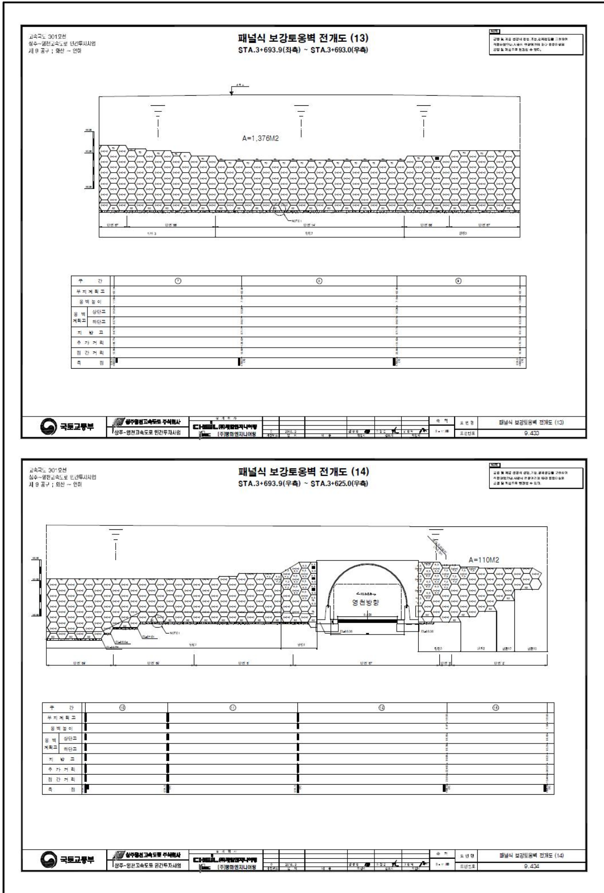
【그림 15.4】전개도(계속)
